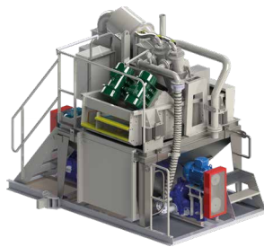
D120-50 Dessableur double cyclonage 120 m 3 /h au primaire 50 m 3 /h au secondaire
