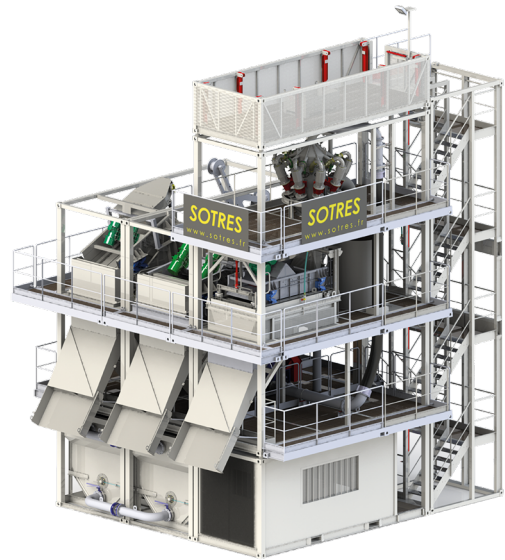
D500-500 Dessablage avec scalpage + double cyclonage 500 m 3 /h au primaire 500 m 3 /h au secondaire
