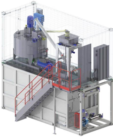
Préparateur à bentonite
